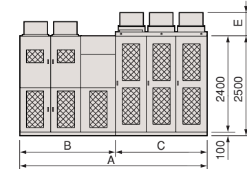
Fig. 10 6kV: 3200kVA
