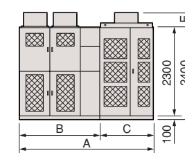
Fig. 7 6kV: 1200, 1400kVA
