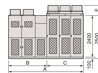
Fig. 9 6kV: 2360, 2700kVA
