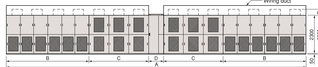
Fig. 13 6kV: 9500kVA
