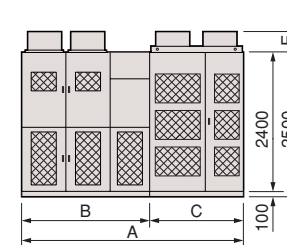
Fig. 8 6kV: 1600, 1800, 2100kVA
