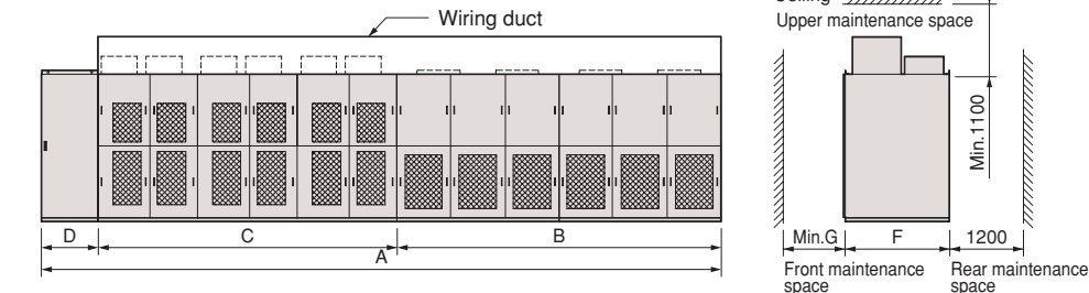
Fig. 25 3kV: 4750kVA
