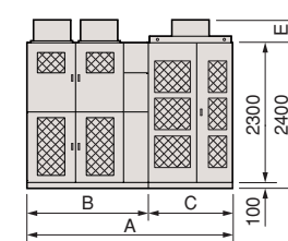
Fig. 6 6kV: 860, 1000kVA
