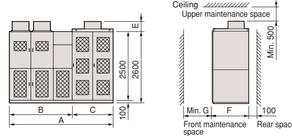
Fig. 15 4.16kV: 1100, 1450kVA
